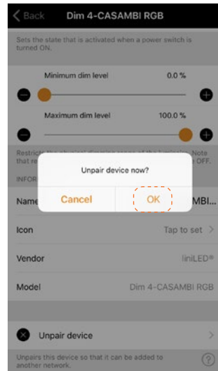
10. Press OK
